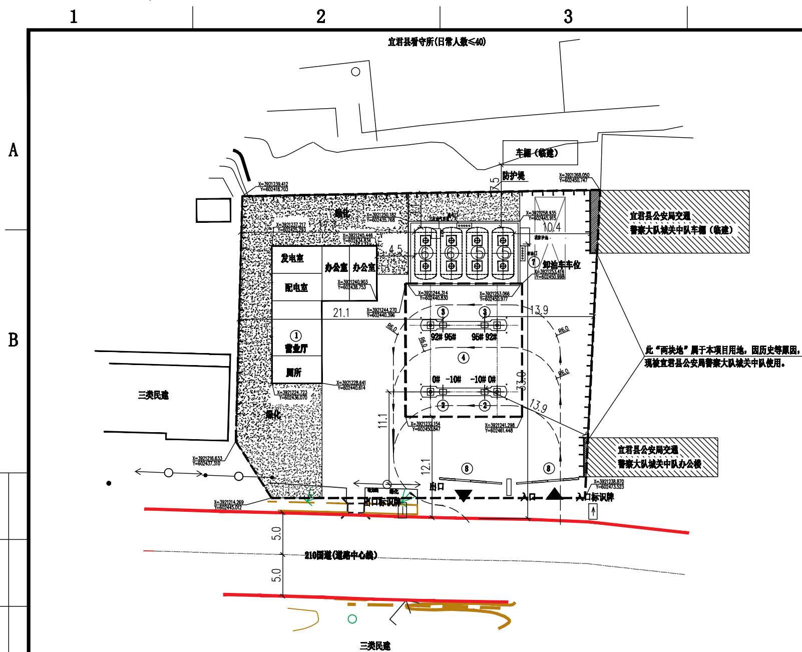
加油站内设施内部建构筑物防火间距表
